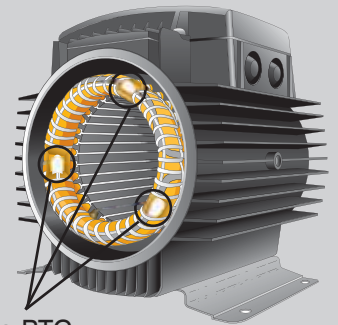
3 датчика ПТК; По одному на каждой фазе
