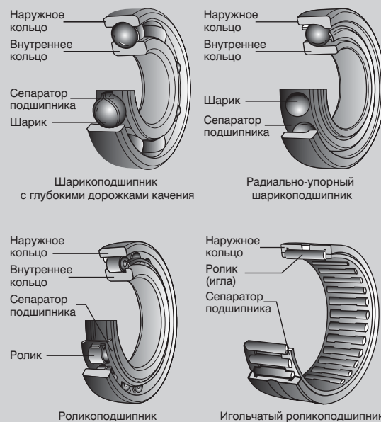
Различные типы шариковых и роликовых подшипников
