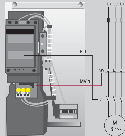
K 1 = Контактор MV 1 = Реле перегрузки
