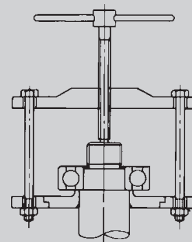
Выпрессовка подшипника
