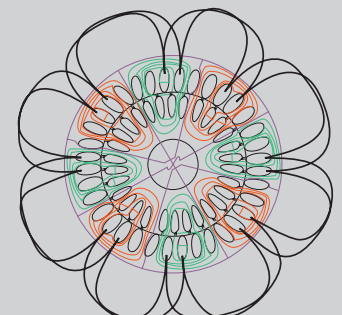
3-фазный, 8-полюсный электродвигатель
