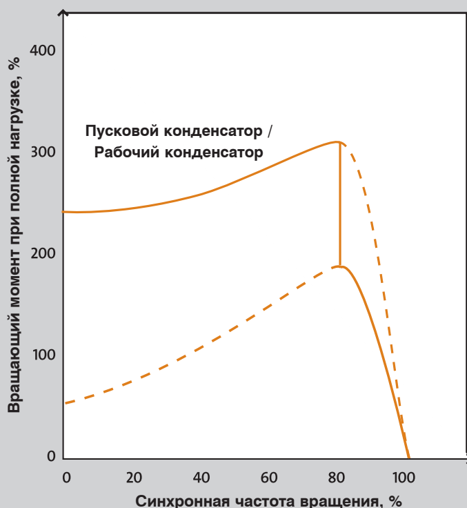
Электродвигатель CSCR. Схема электрических соединений и характеристика пусковой момент/частота вращения
