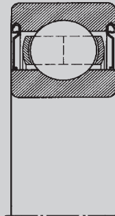
Шарикоподшипник с глубокими дорожками качения с металлическими стыковыми накладками. Известен как тип ZZ
