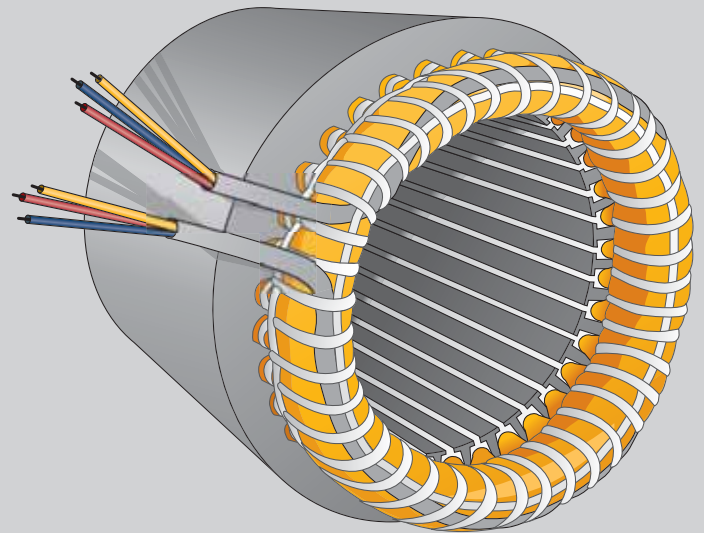
Статор
