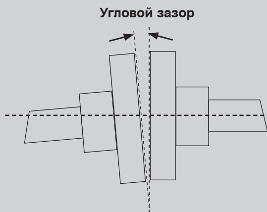
Угловое выравнивание
