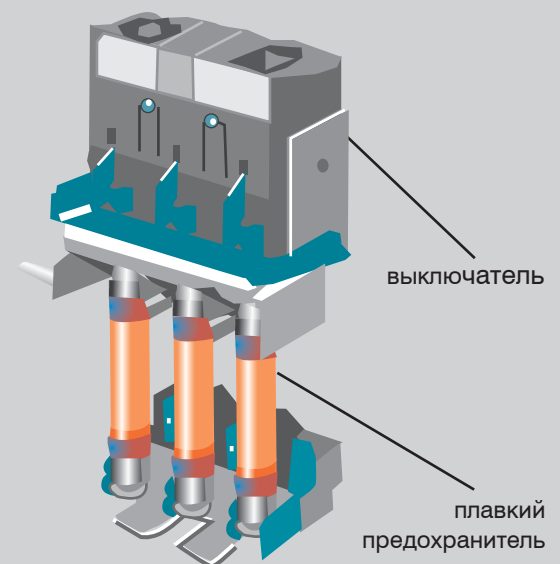
Плавкий предохранительный выключатель
