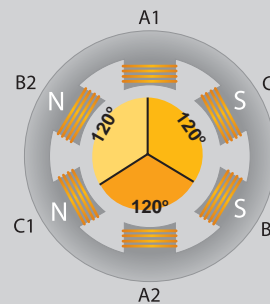
Обмотки фаз и число полюсов
