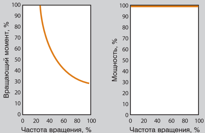
При увеличении скорости вращения уменьшается вращающий момент, при этом мощность остаётся постоянной
