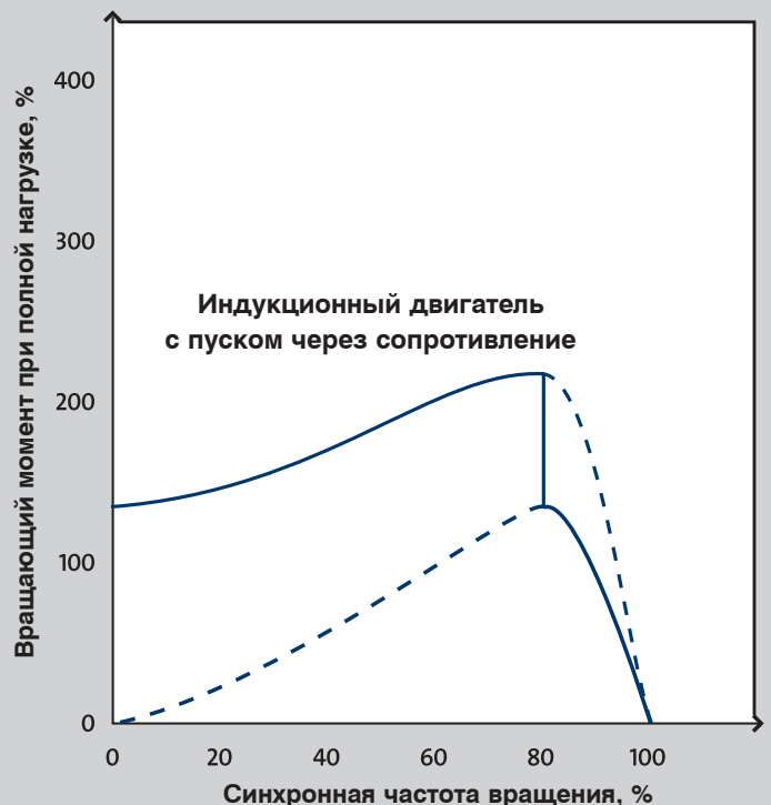
Электродвигатель RSIR. Схема электрических соединений и характеристика пусковой момент/частота вращения
