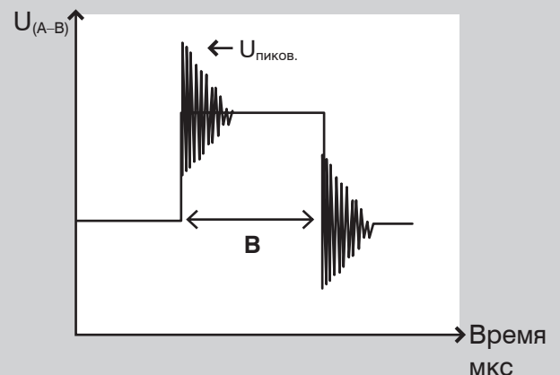
Выходной импульс с U_{\text{пиков.}} .
