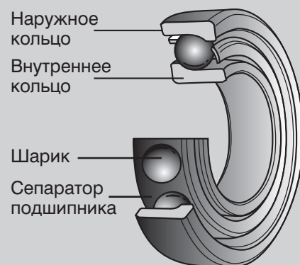
Радиально-упорный шарикоподшипник
