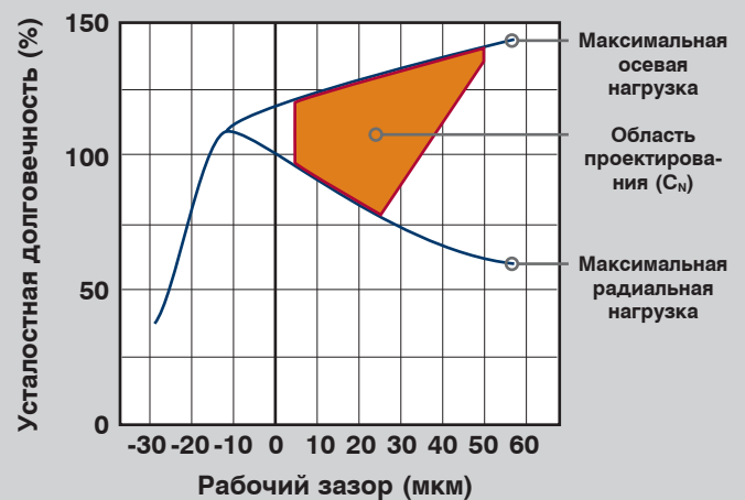
Соотношение между долговечностью и рабочим зазором для шарикоподшипников с глубокими дорожками
