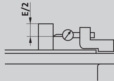
Эксцентricность вала электродвигателей В14/В18/В5/В1
