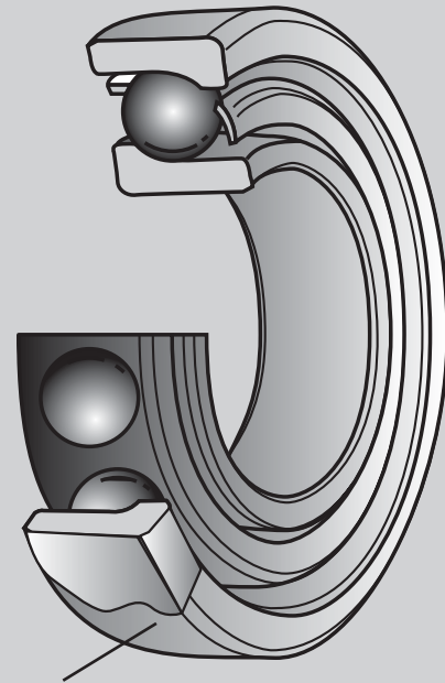
Керамический слой
