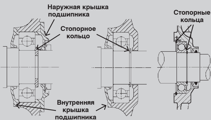
Схема установки зафиксированных DE-подшипников
