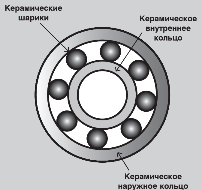
Полностью керамические подшипники
