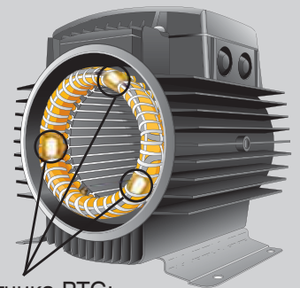
Три датчика РТС: по одному в каждой фазе
