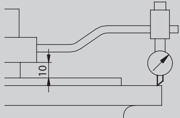
Перпендикулярность установочной поверхности фланца к валу
