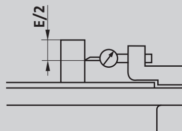
Эксцентриситет конца вала для электродвигателей В14/В18/В5/В1
