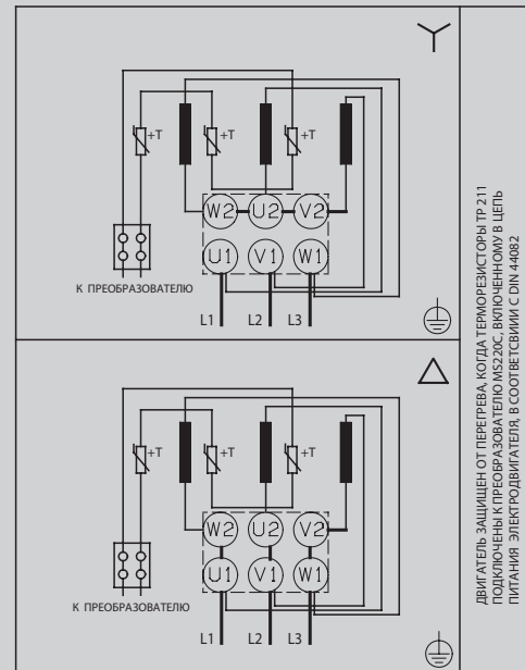
Типичная схема электрических соединений
