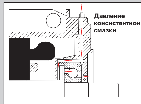
Конструкция смазочной системы
