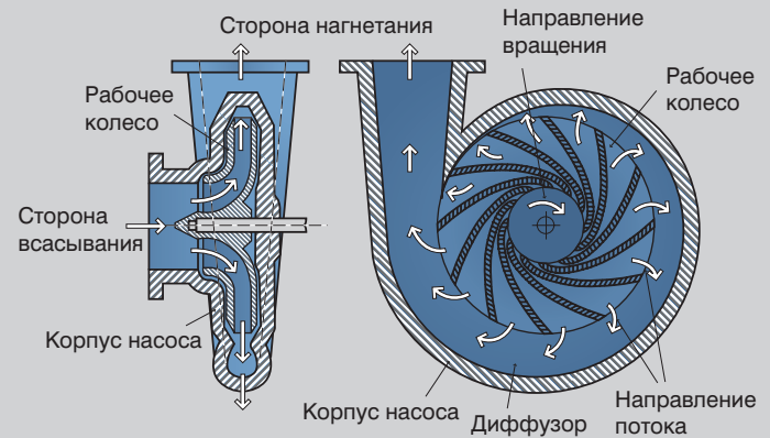
Центробежный насос, поперечный разрез
