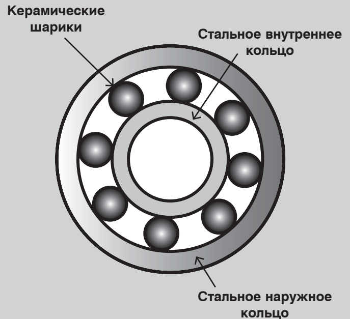
Гибридные подшипники
