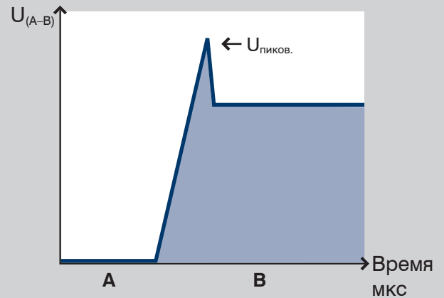
Упрощённый выходной импульс с U_{\text{пиков.}} .
