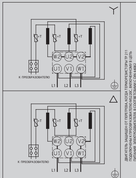
Схема подключения
