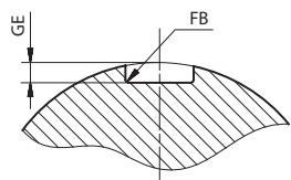
Сторона присоединения привода
