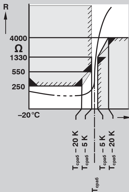
Сопротивление в зависимости от температурной характеристики терморезистора PTC (DIN 44081/44082)
