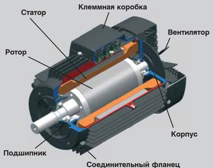
Электродвигатель
