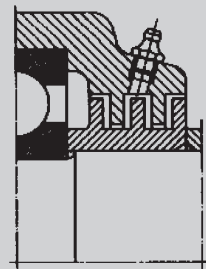
Лабиринтное уплотнение
