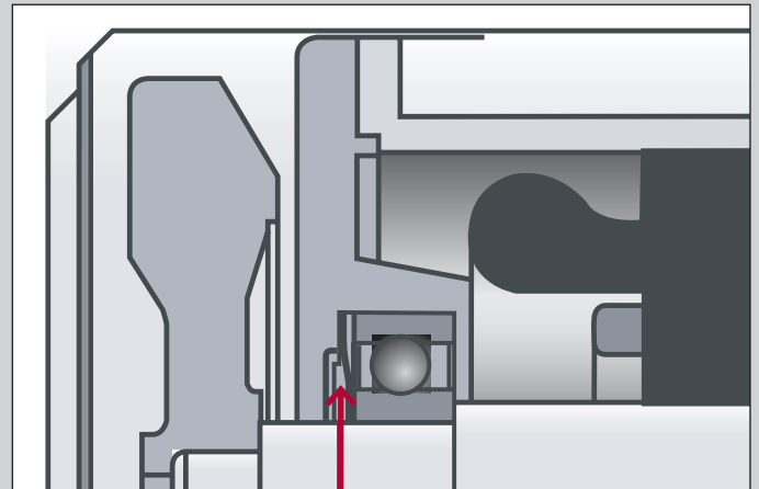
Пружина, обеспечивающая предварительный натяг
