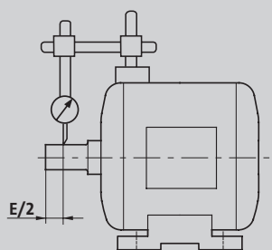
Электродвигатели с эксцентриситетом конца вала В3
