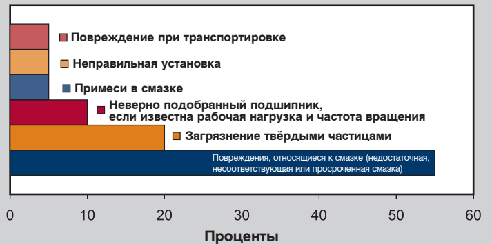
Причины разрушения подшипников качения
