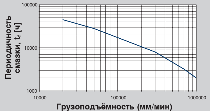
Базовая периодичность смазки
