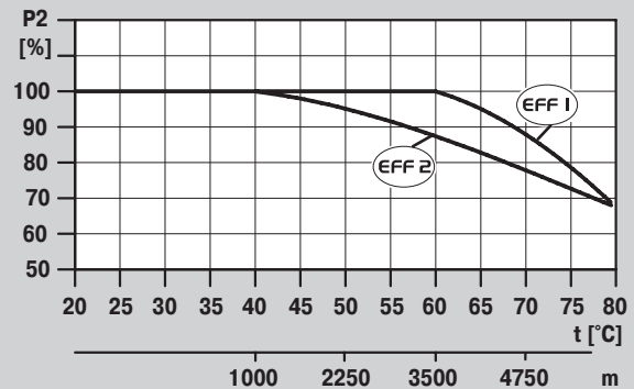
Кривая понижения выходной мощности с ростом температуры окружающей среды или увеличением высоты установки над уровнем моря
